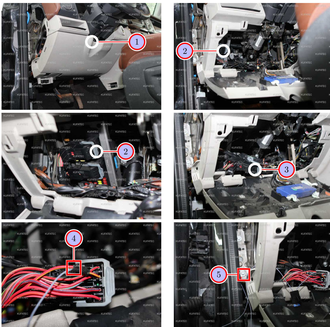
Abbildung 5: Anschluss Zündungsplus / Masse
