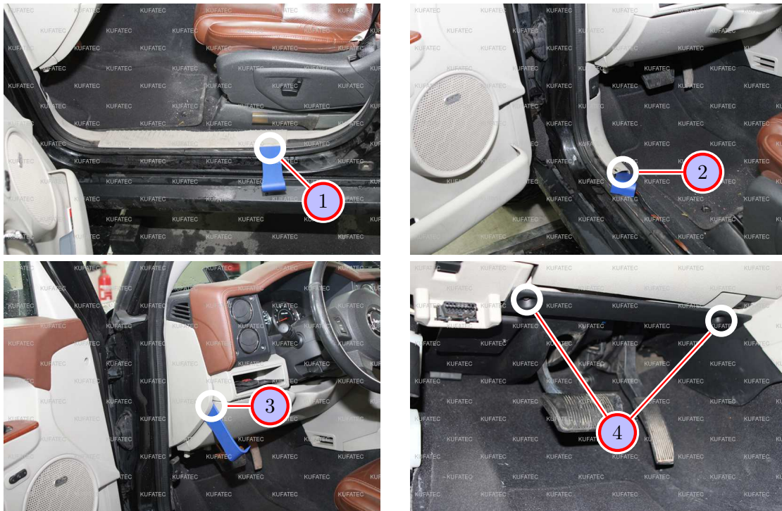
Abbildung 4: Demontage Verkleidung Fahrerseite
