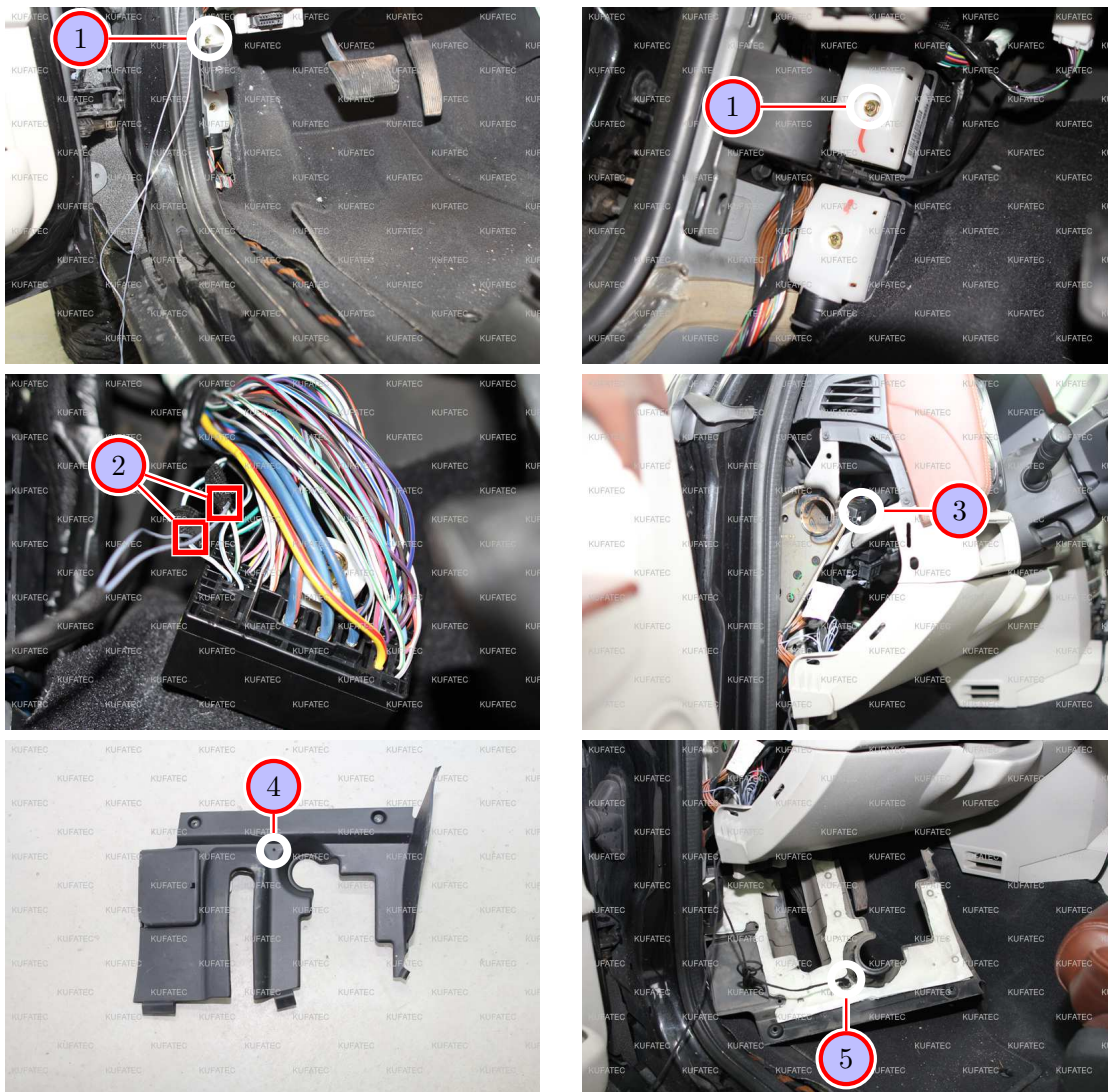
Abbildung 6: Anschluss Can High & Low / Montage Taster
