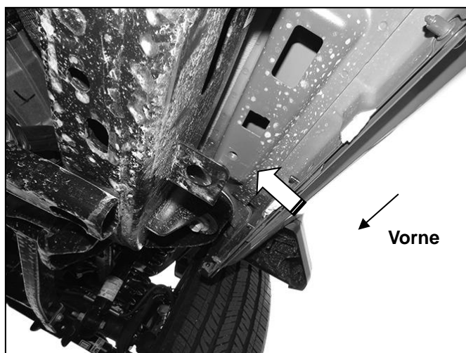
(Bild 2) Vorderer Montagepunkt mit Innengewinde auf der Beifahrerseite/Rechts
