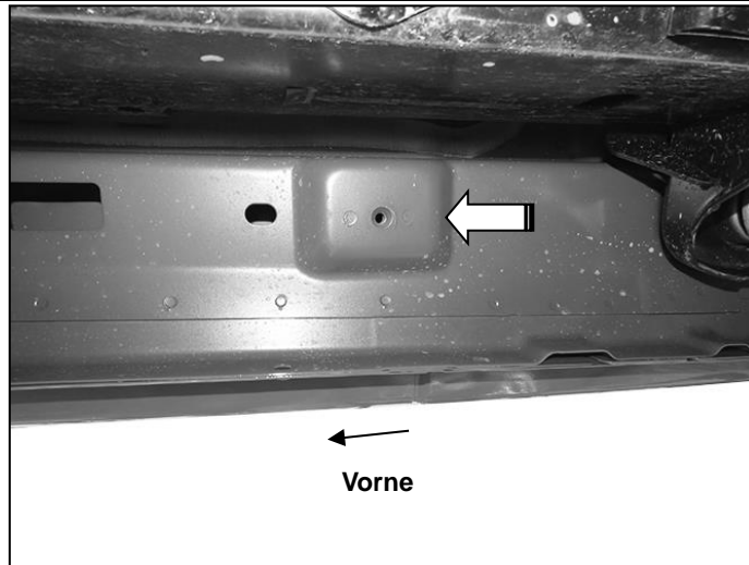
(Bild 3) Zweiter Montagepunkt Beifahrerseite/Rechts
